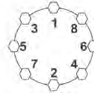
8-Lug Nuts
